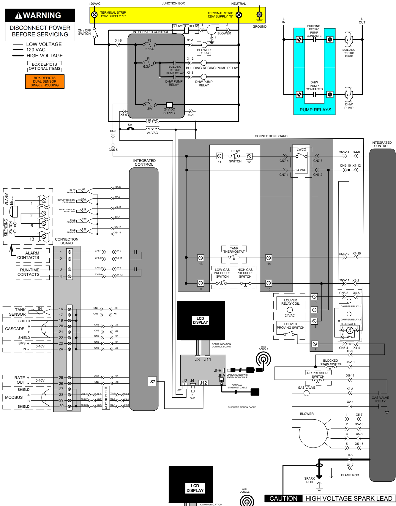
Figure 14-1 Schéma électrique
