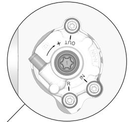
Figure 2-4 Réglage de la vanne du gaz: modèles 650 - 1000 Séries 110 - 111
