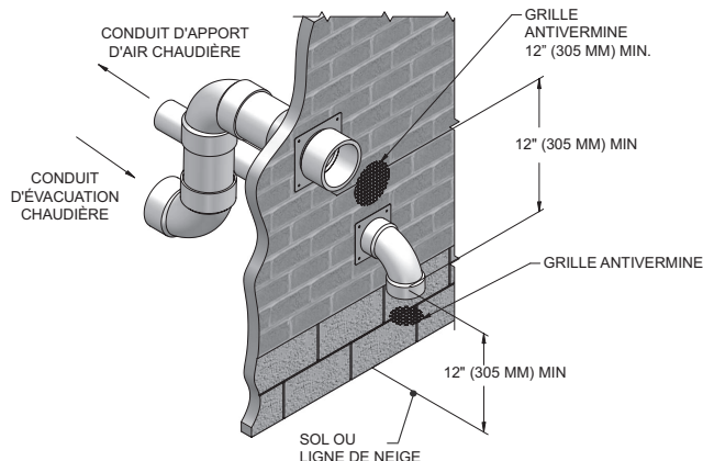
Figure 4-2 Terminaisons murales optionnelles en PVC/CPVC/inox./polypropylène (non fournies)
