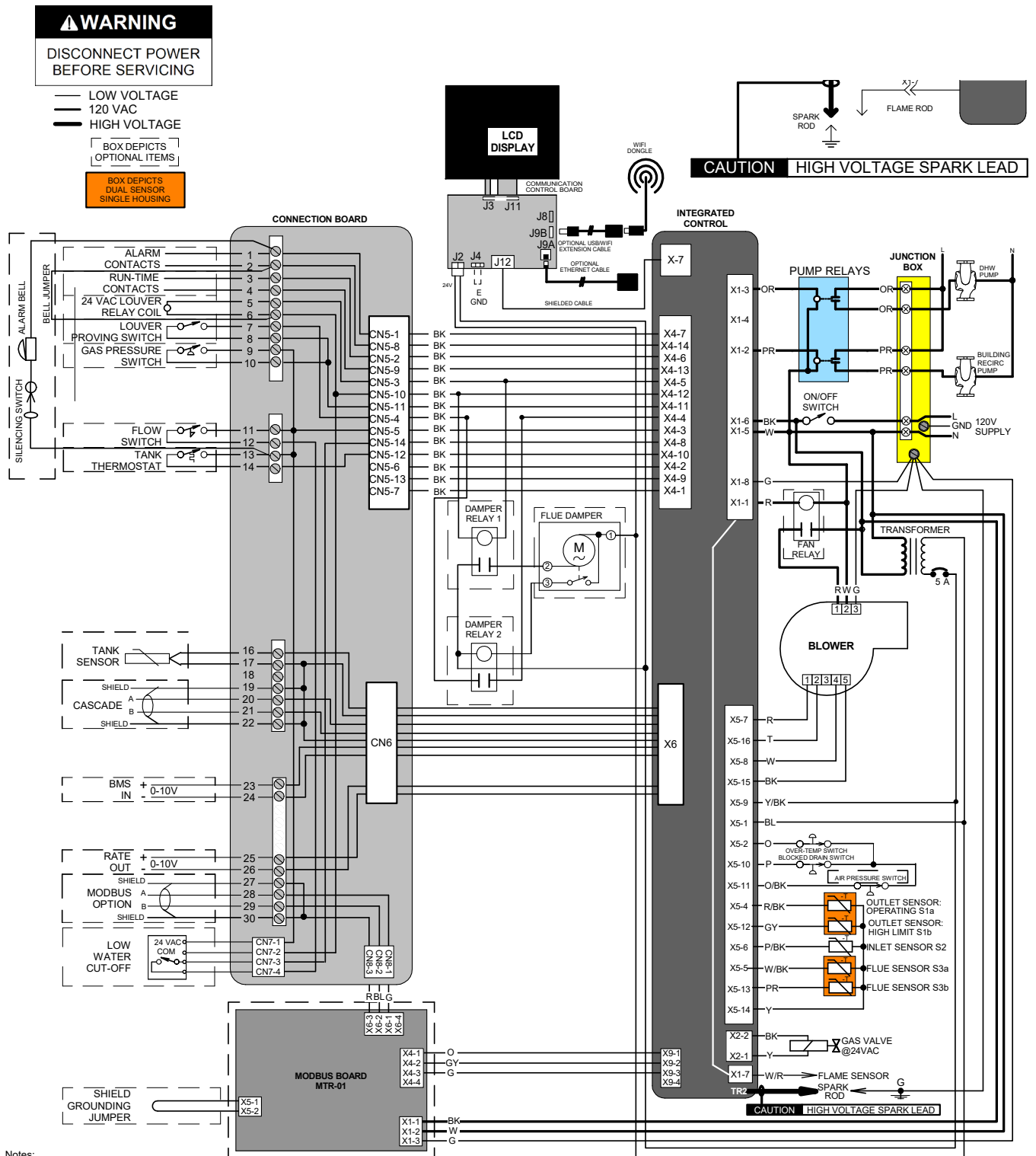
Figure 14-2 Schéma de câblage
