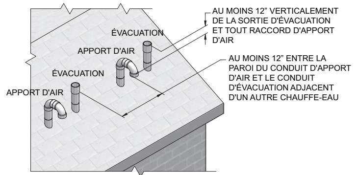
Figure 5-2 Terminaisons verticales, plusieurs chauffe-eau
