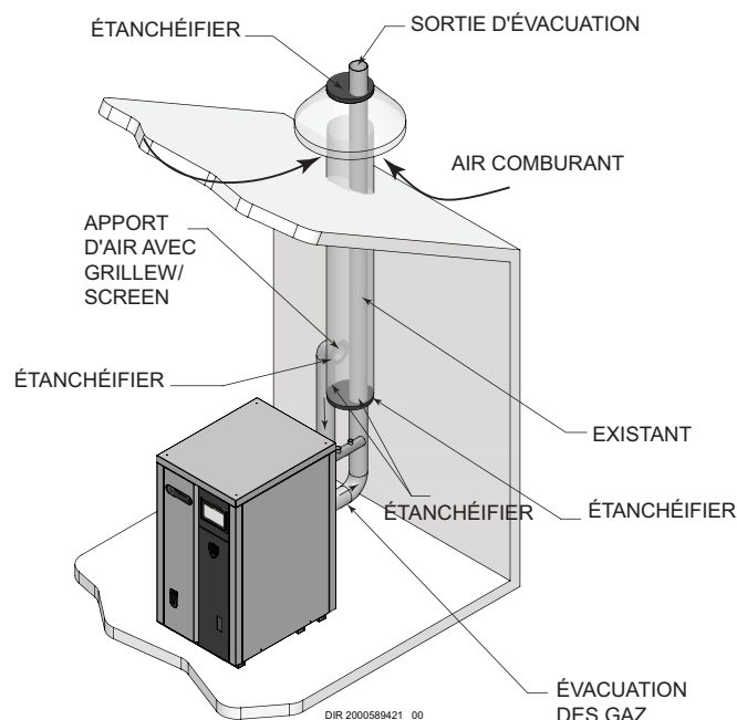
Figure 5-9 Ventilation concentrique, exemple 2
