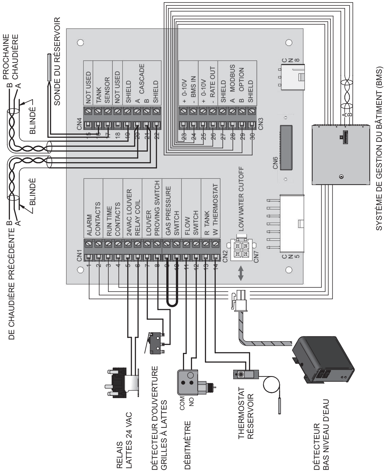
Figure 9-3 Raccords basse tension au chantier
