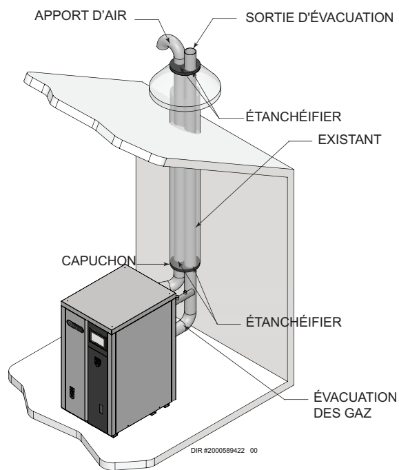
Figure 5-10 Utilisation d'un passage existant
