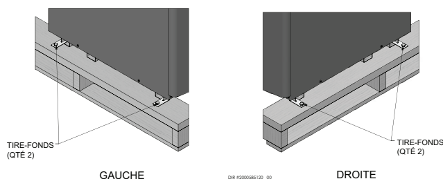
Figure 2-1 Chauffe-eau monté sur sa palette d'expédition
