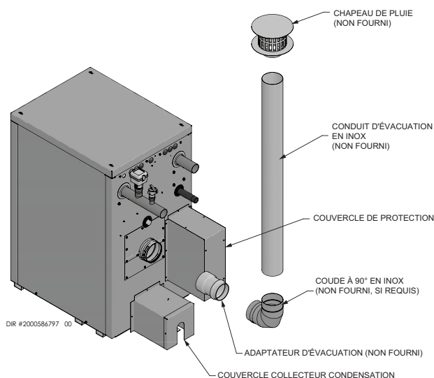
Figure 6-2 Ventilation extérieure, acier inoxydable
