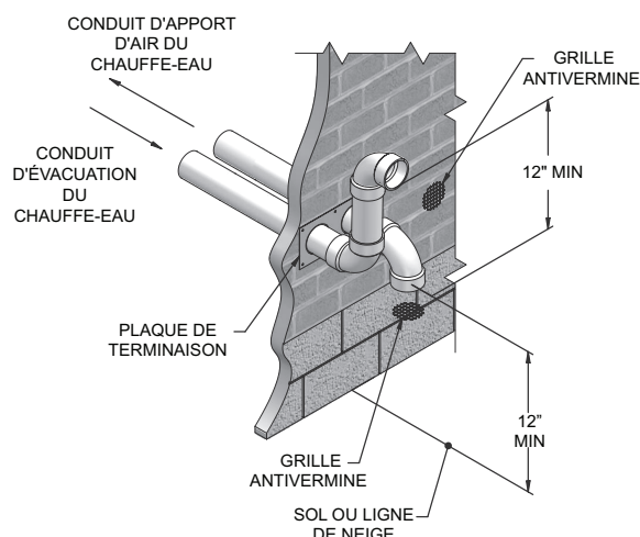
Figure 4-1B Terminaisons d'apport d'air et d'évacuation murales optionnelles en PVC/CPVC (non fournies)
